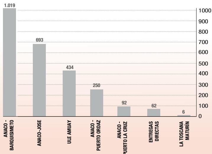
GRÁFICO • VOLUMEN MANEJADO POR SISTEMAS DE TRANSPORTE 2.556 MMPCD
