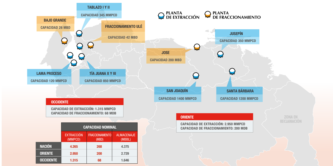
GRÁFICO • INFRAESTRUCTURA DE PROCESAMIENTO DE LGN
