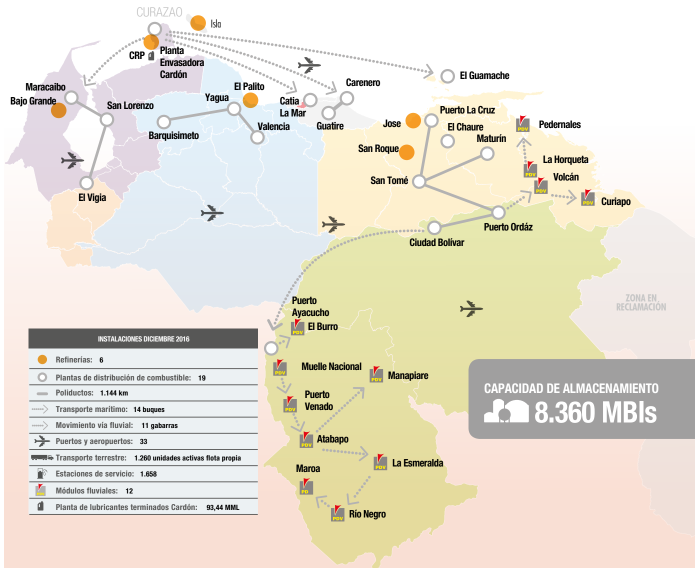
GRÁFICO • SISTEMA DE TRANSPORTE, ALMACENAMIENTO Y DISTRIBUCIÓN
