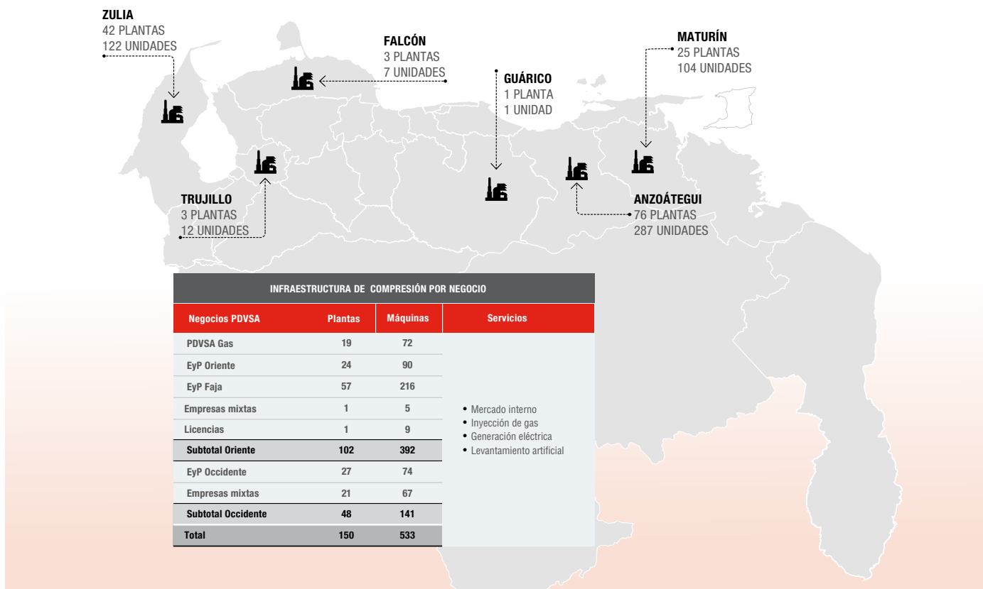
GRÁFICO • INFRAESTRUCTURA DE COMPRESIÓN
